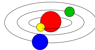
GRAVEDAD
