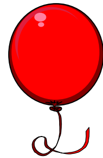
AIRE/GAS
